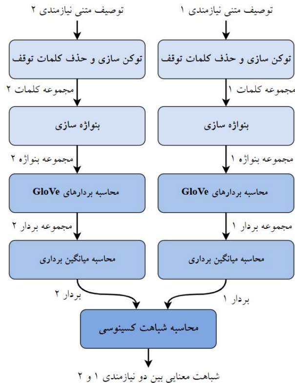
شکل (3): نحوه محاسبه شباهت معنایی بین نیازمندی‌ها
