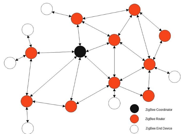
شکل (۹): شبکه ZigBee
