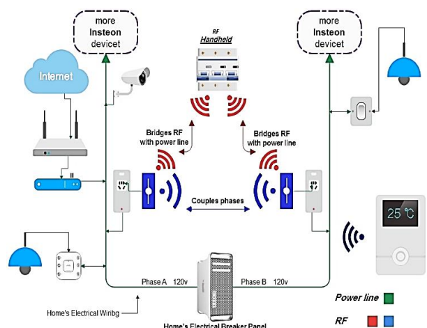
شکل (۳): ساختار شبکه INSTEON
