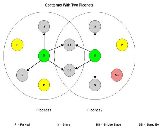
شکل (۸): معماری شبکه فناوری بلوتوث
