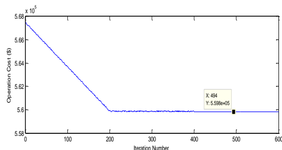
شکل (۴): مشخصه همگرایی الگوریتم پیشنهادی در شبکه شامل ۱۰ واحد
