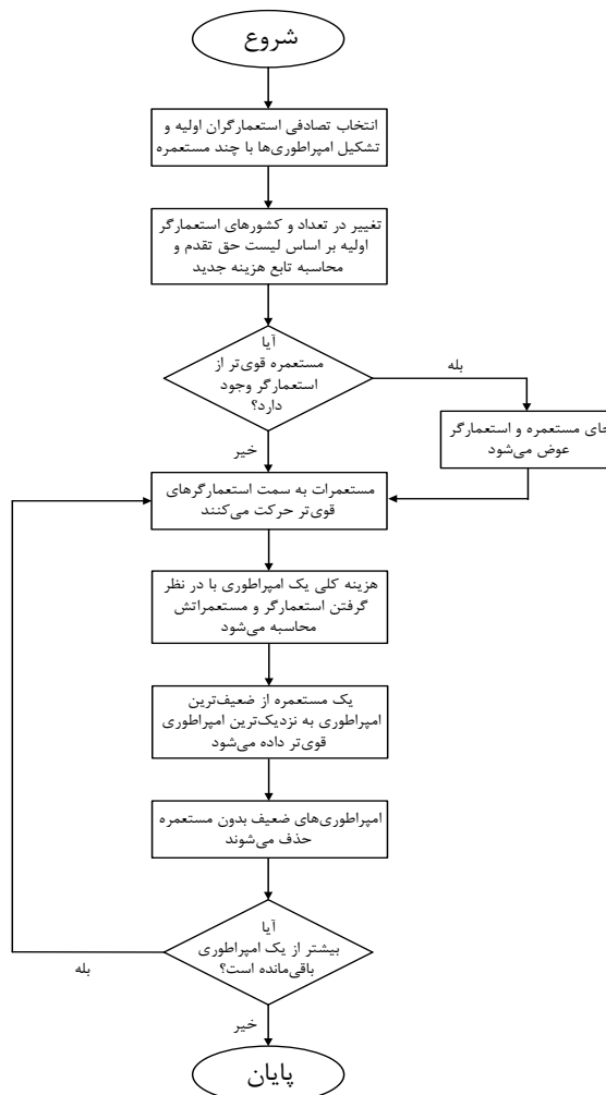
شکل (۳): فلوچارت الگوریتم بهینه‌سازی رقابت استعماری اصلاح شده
