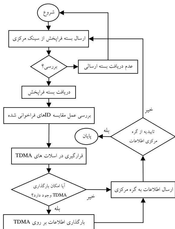
شکل (۸): فلوجارت یک فریم ارسالی در پروتکل پیشنهادی
