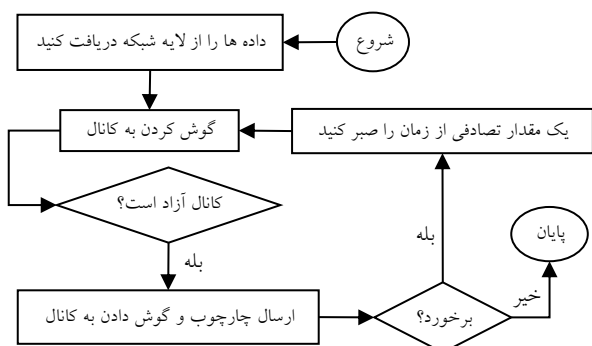
شکل (۵): پروتکل CSMA [۱]
