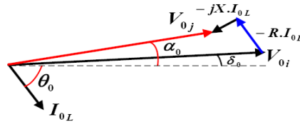
شکل (3): دیاگرام فازوری ولتاژها و جریان‌های شکل (2)
