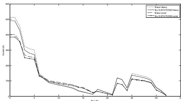
شکل (10): پروفیل جریان قبل و بعد از جایگذاری DSTATCOM در
