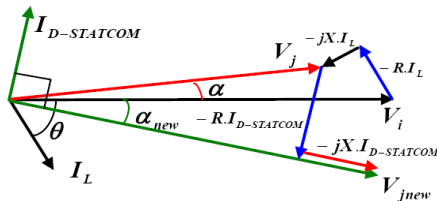
شکل (5): دیاگرام فازوری ولتاژها و جریان‌های شبکه شکل (4)
